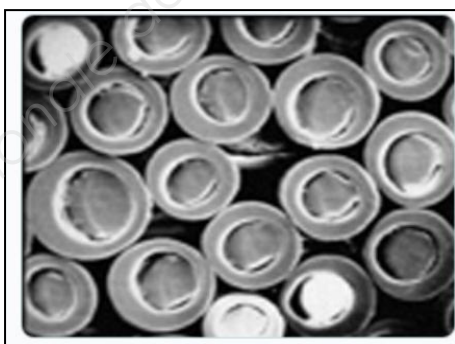
Fibres polyester au microscope Nouveau procédé de filature, cœur en PCM et enveloppe en polyester.
