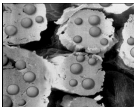
Fibres acryliques avec capsules PCM Très résistant à l'abrasion et aux rayons solaires – séchage rapide.
